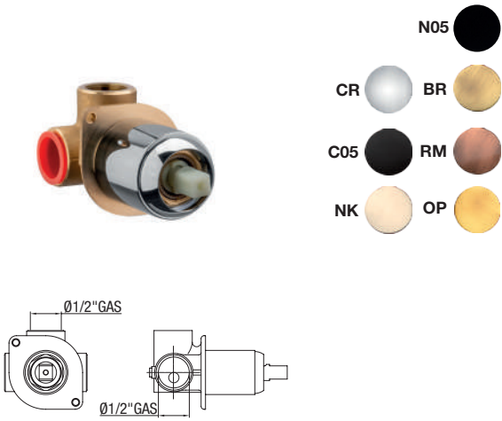
FR 25 CL Corpo incasso doccia Built-in shower body Corps pour douche à encastrer
