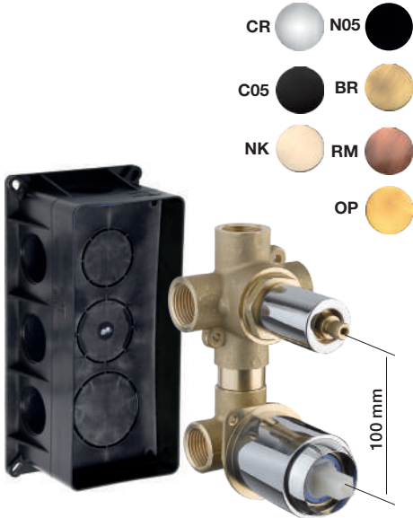
FR3V-S 3 vie con scatola incasso 3 ways with built-in wall box 3 voies avec boîte à encastrer
