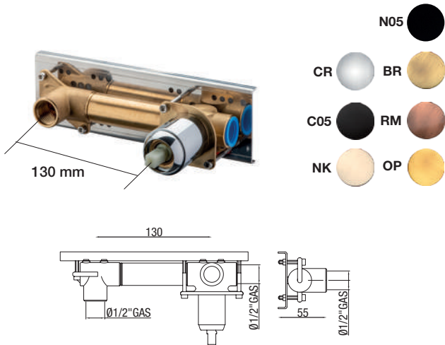
FR LI 25 CL Corpo miscelatore incasso lavabo Built-in basin mixer Corps de mitigeur pour lavabo
