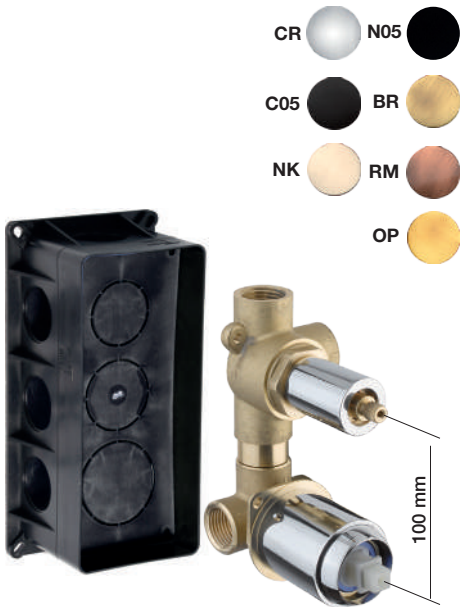
FR2V-S 2 vie con scatola incasso 2 ways with built-in wall box 2 voies avec boîte à encastrer
